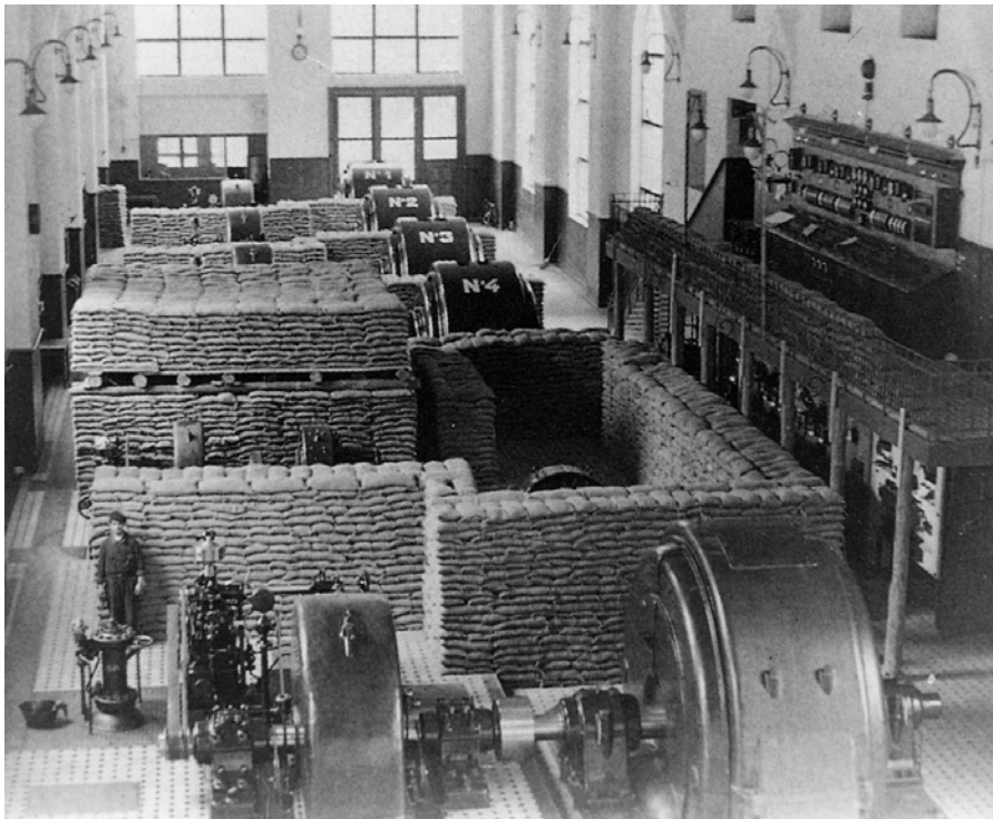
Estació receptora de la central de Talarn protegida amb sacs terrers. Generadors de la central de Cabdella, protegits amb sacs terrers l'any 1937. Arxiu: Fons històric d'Endesa.
